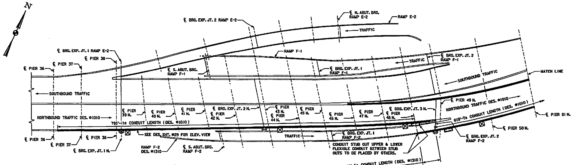
CONDUIT LAYOUT PLAN
